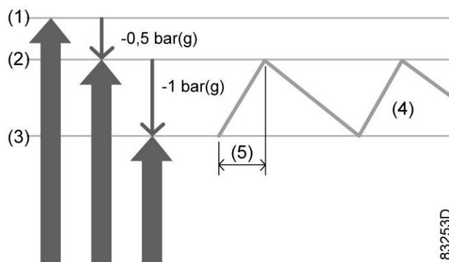
Исполнения с измерением в %: установки для уровней Давления останова и Давления пуска
