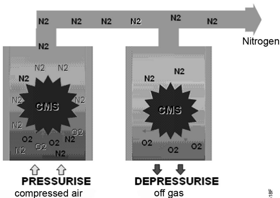
Принцип работы генератора азота
