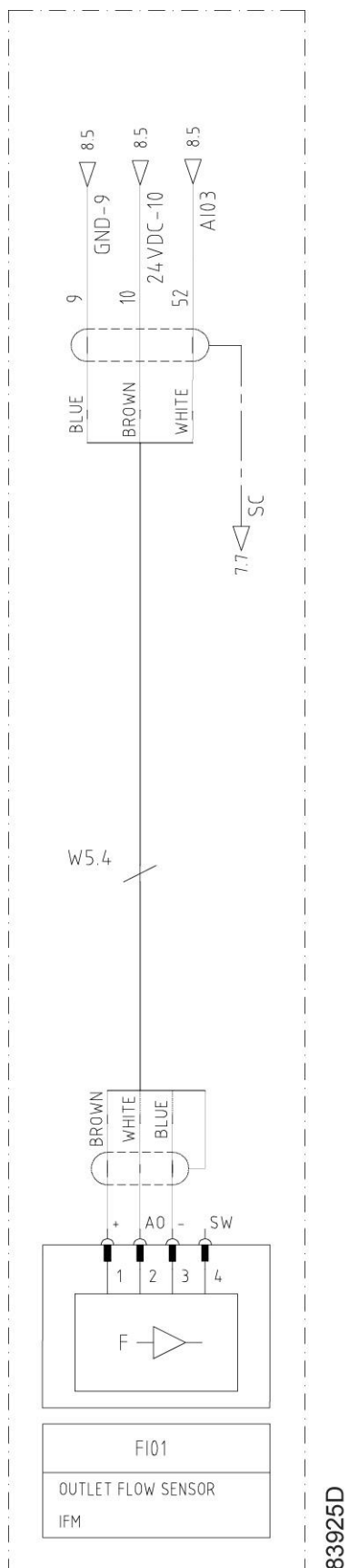
Электрическая схема подключения датчика расхода IFM - PPNG-1.5-150 PCT, PPNG-1.5-540 PPM (9827 2664 00)
