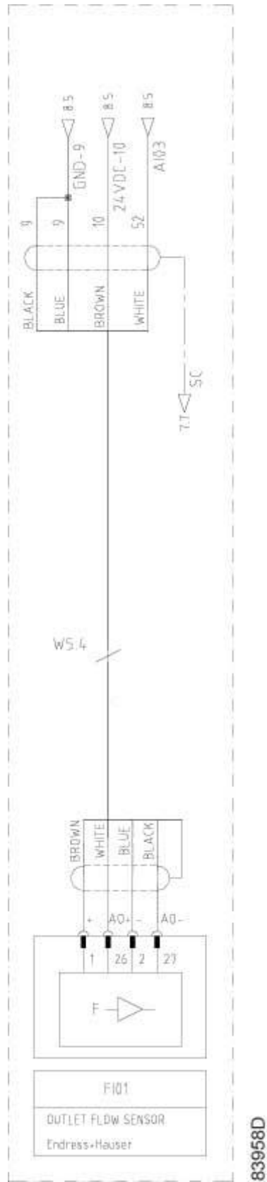
Электрическая схема подключения датчика расхода Endress+Hauser - PPNG-250-650 PCT, PPNG-650 PPM (9827 2664 00)
