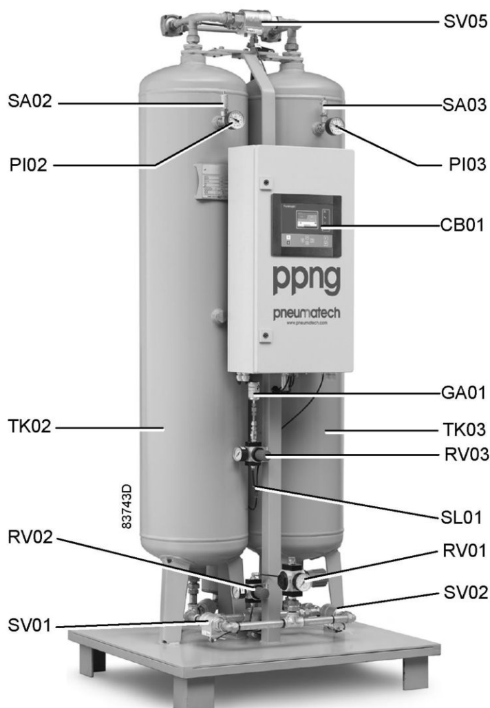
PPNG-9, вид спереди
