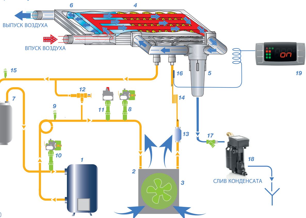
СХЕМА CDX 240
