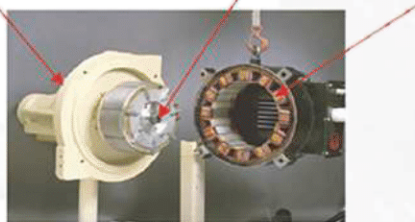
Статор двигателя
